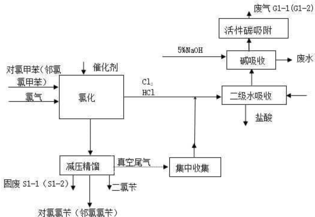
图 4.1-1 对氯氯苯（邻氯氯苯）项目工艺流程图
