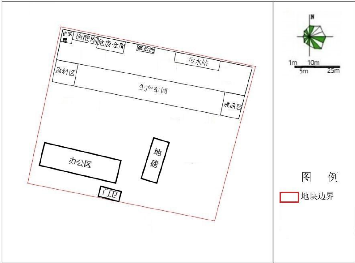
图2.1-2 厂区平面布置图
